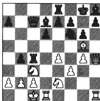
na 20. ..., b4!
