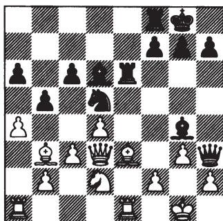
na 18. a2-a4
