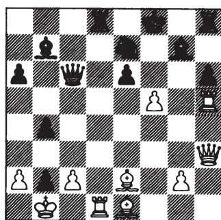
na 29. Ke1-b1
