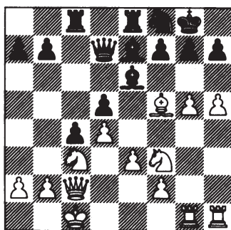
na 17. ..., Dd8-d7
