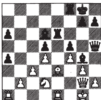
na 22. Df1-g2
