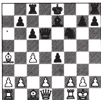
na 12. ..., Lf8-e7
