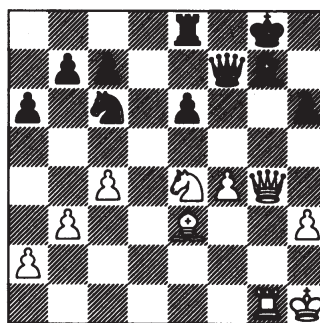
na 27. ..., Df6-f7
