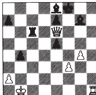
na 34. ..., Tc6
