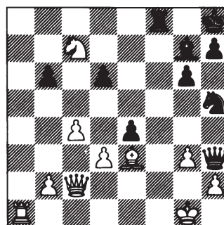
na 25. Pd5xc7
