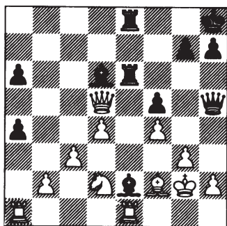
na 25. Kg1-g2!
