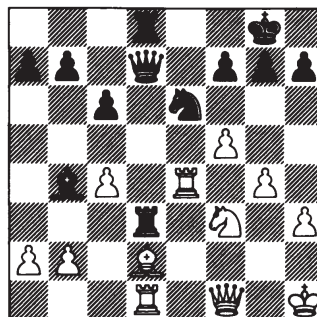
na 28. f4-f5
