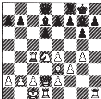
na 16. Pe2
