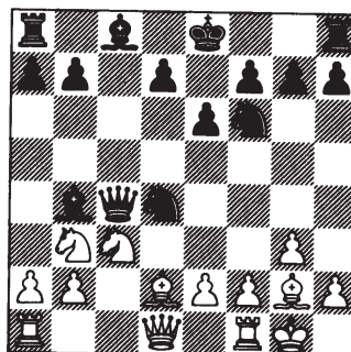
wit aan zet na 10. ..., Pd4
